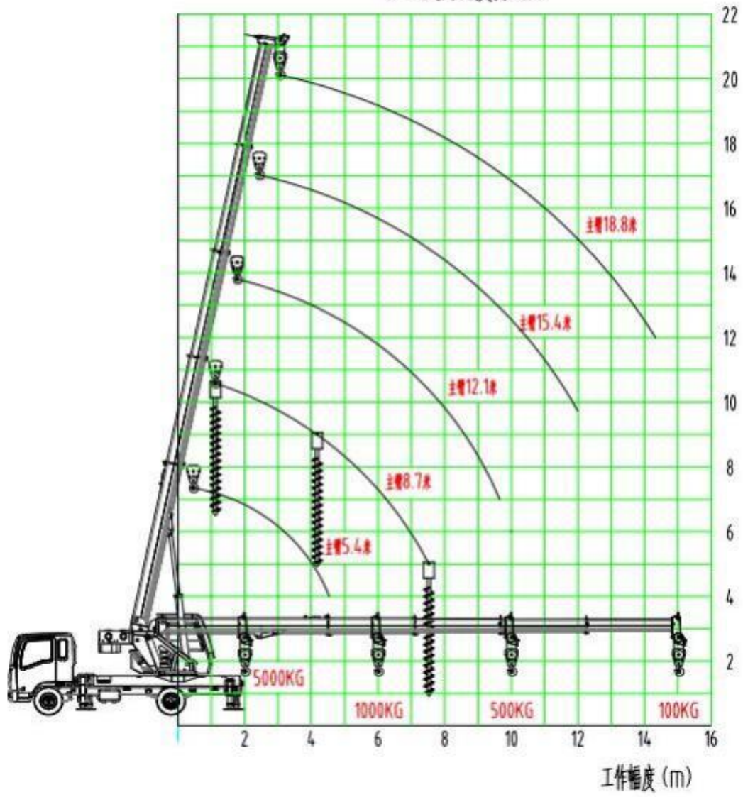
5T.起升高度曲线图
